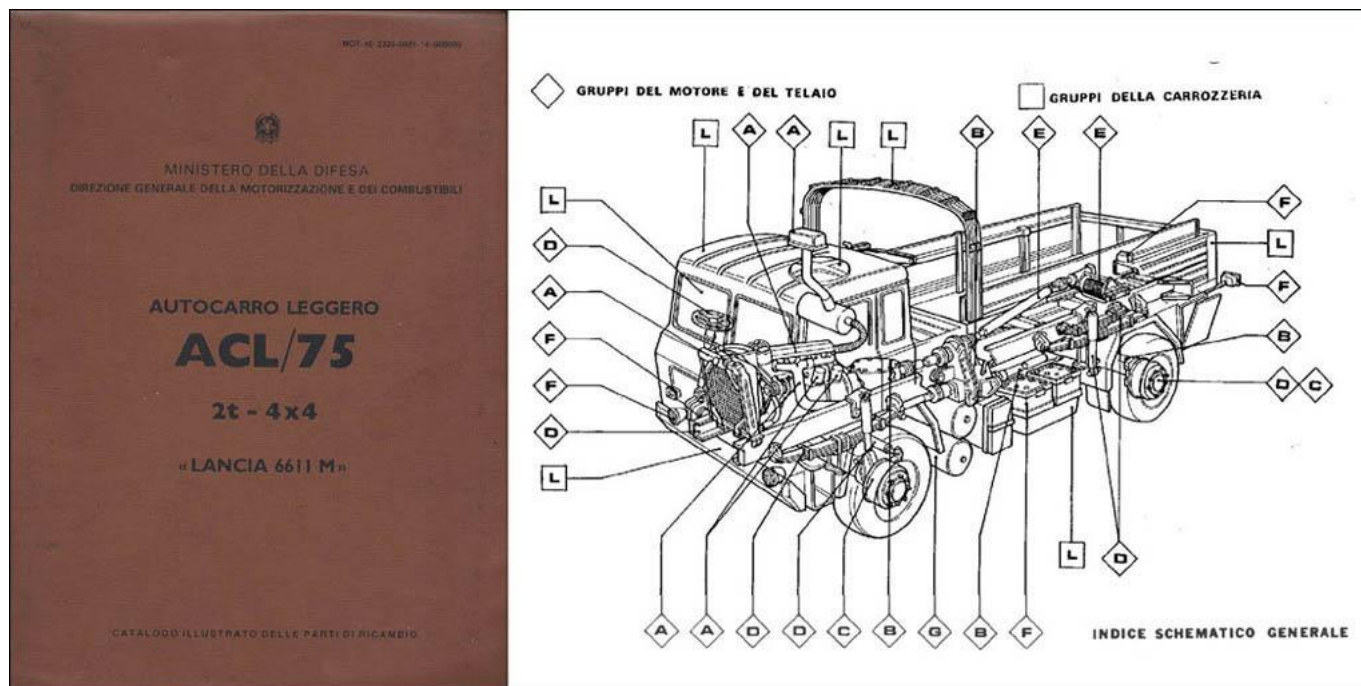
Ministero della Difesa - Autocarro leggero ACL/75 -2t 4x4 - LANCIA 6611 M Catalogo parti di ricambio - pagine 737
