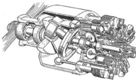
Motore a piatto oscillante
