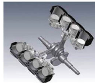
Motore 8 pistoni 2 bielle
